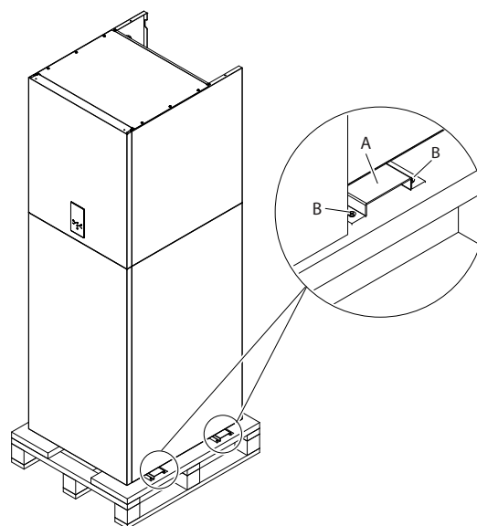
rys. 7 - Jak usunąć wsporniki mocujące
