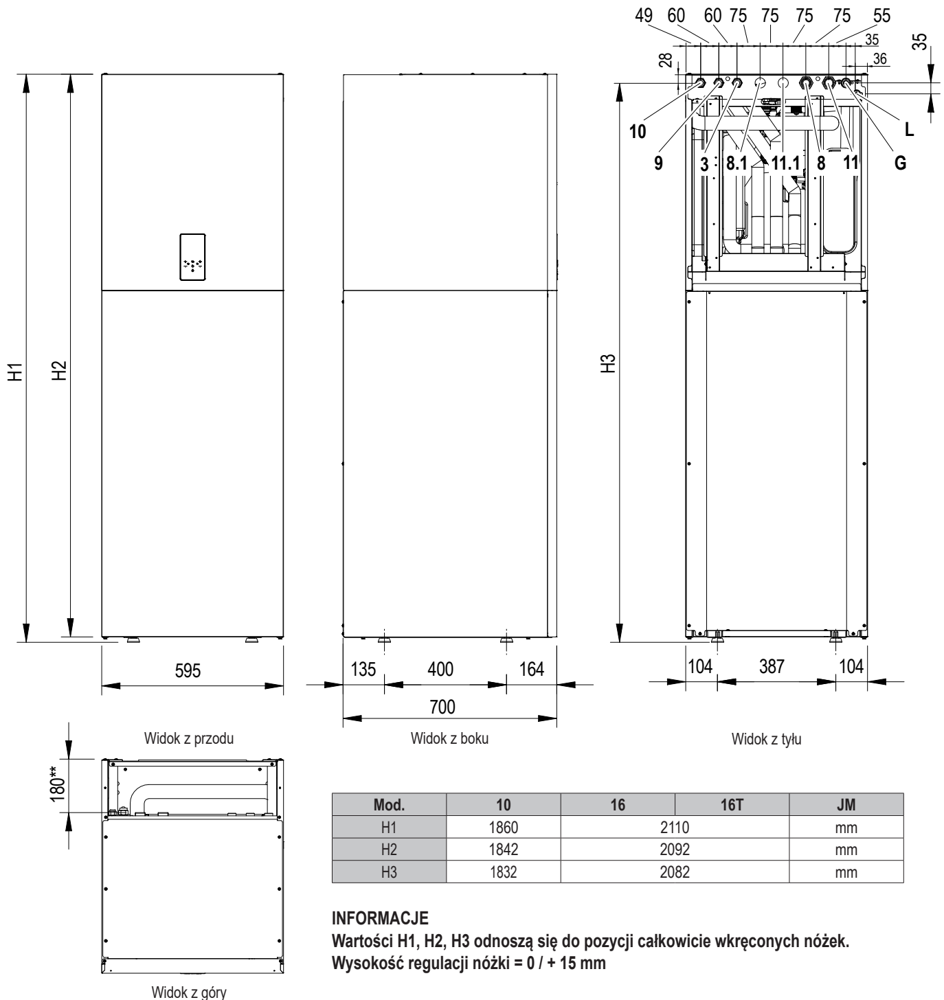
rys. 3 - dane wymiarowe i połączenia
