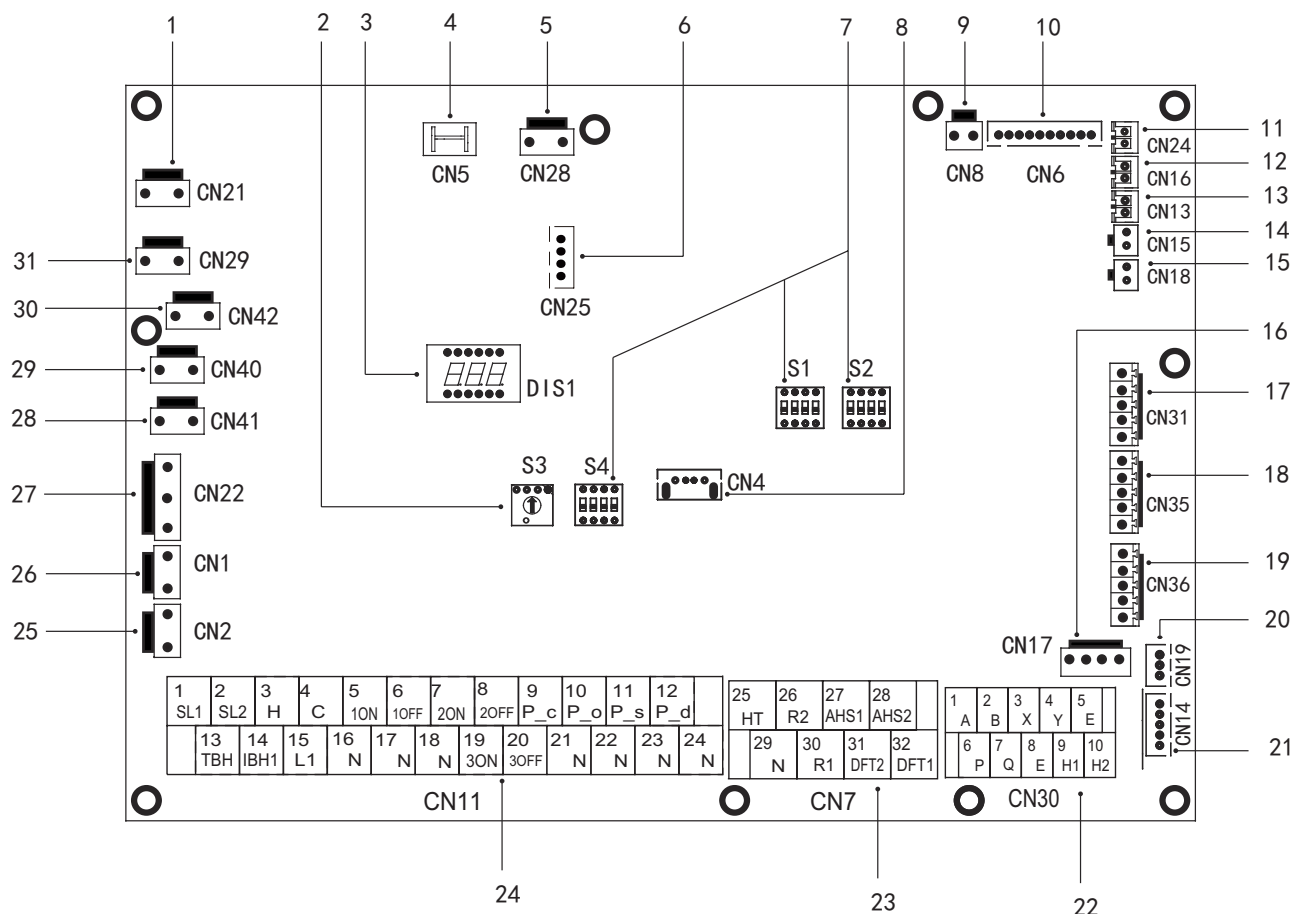
rys. 22 - Płytką systemu wodnego
